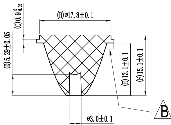
剖面 A-A
